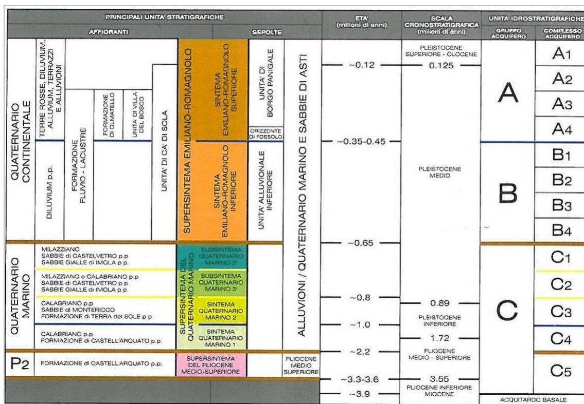
Figura 11 - Schema stratigrafico del margine appenninico e della pianura emiliano romagnola
