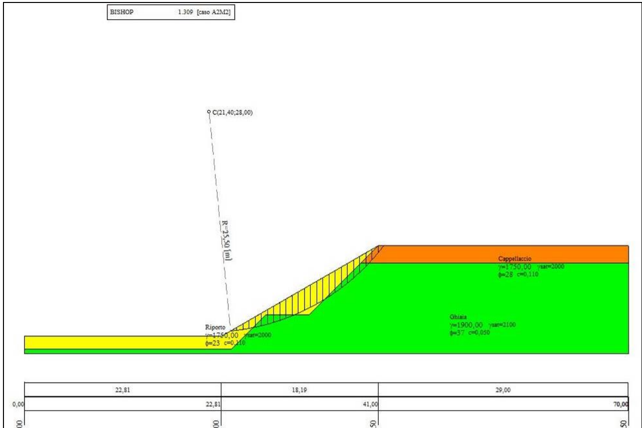
Figura 23 - Geometria di verifica del fronte di sistemazione provvisorio
