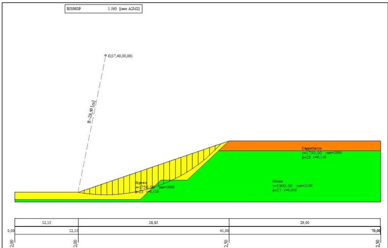
Figura 24 - Geometria di verifica fronte di sistemazione definitivo
